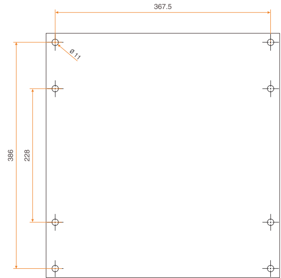
Montaj Şablonu
