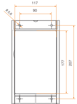
Pano Çerçevesi
