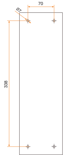
Montaj Şablonu
