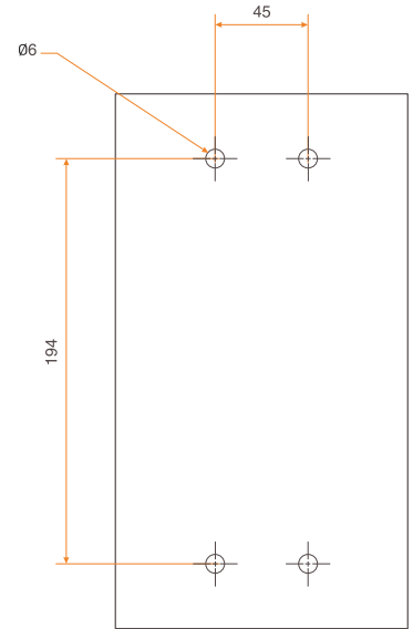
Montaj Şablonu
