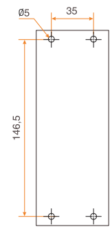
Montaj Şablonu
