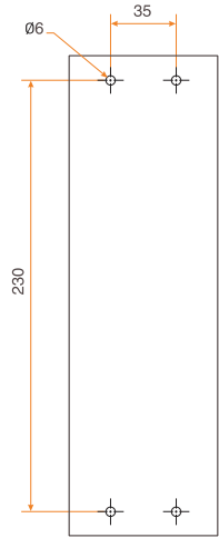
Montaj Şablonu
